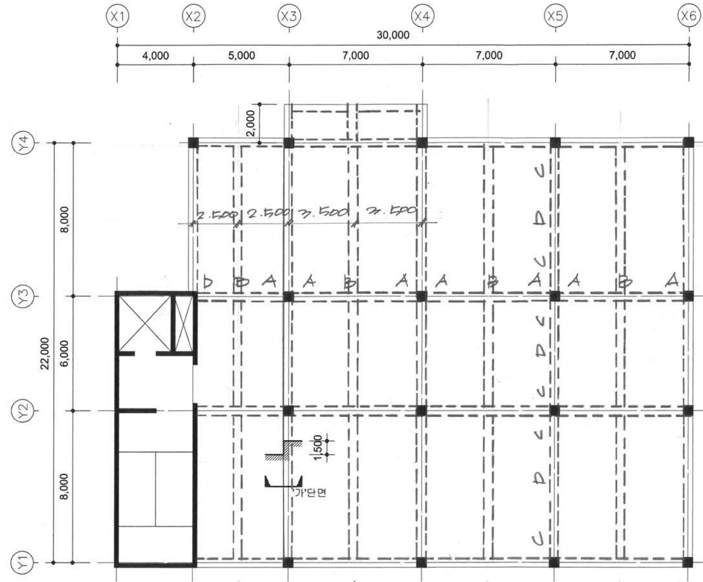
교육동 4층 구조평면도 축척: 1/200
