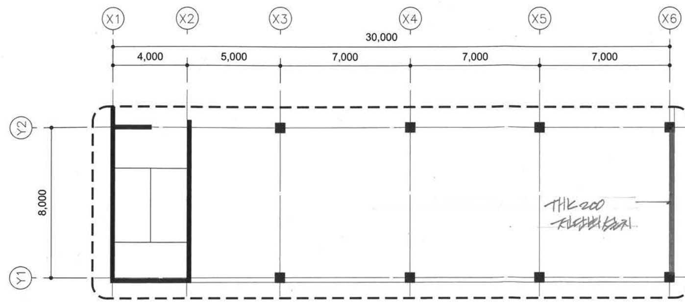
교육동 2층 구조평면도 축척: 1/200
