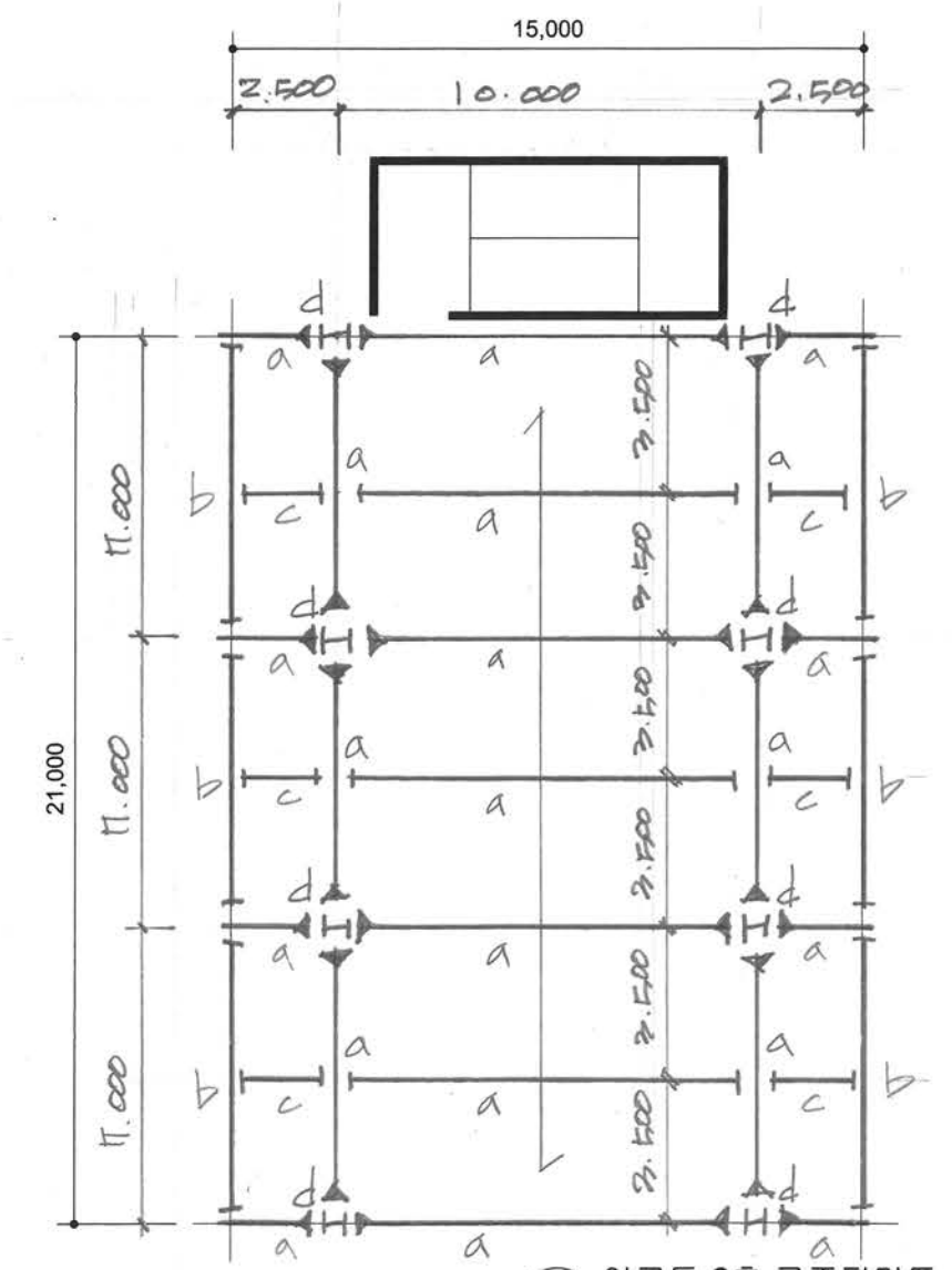
연구동 2층 구조평면도 축척: 1/200
