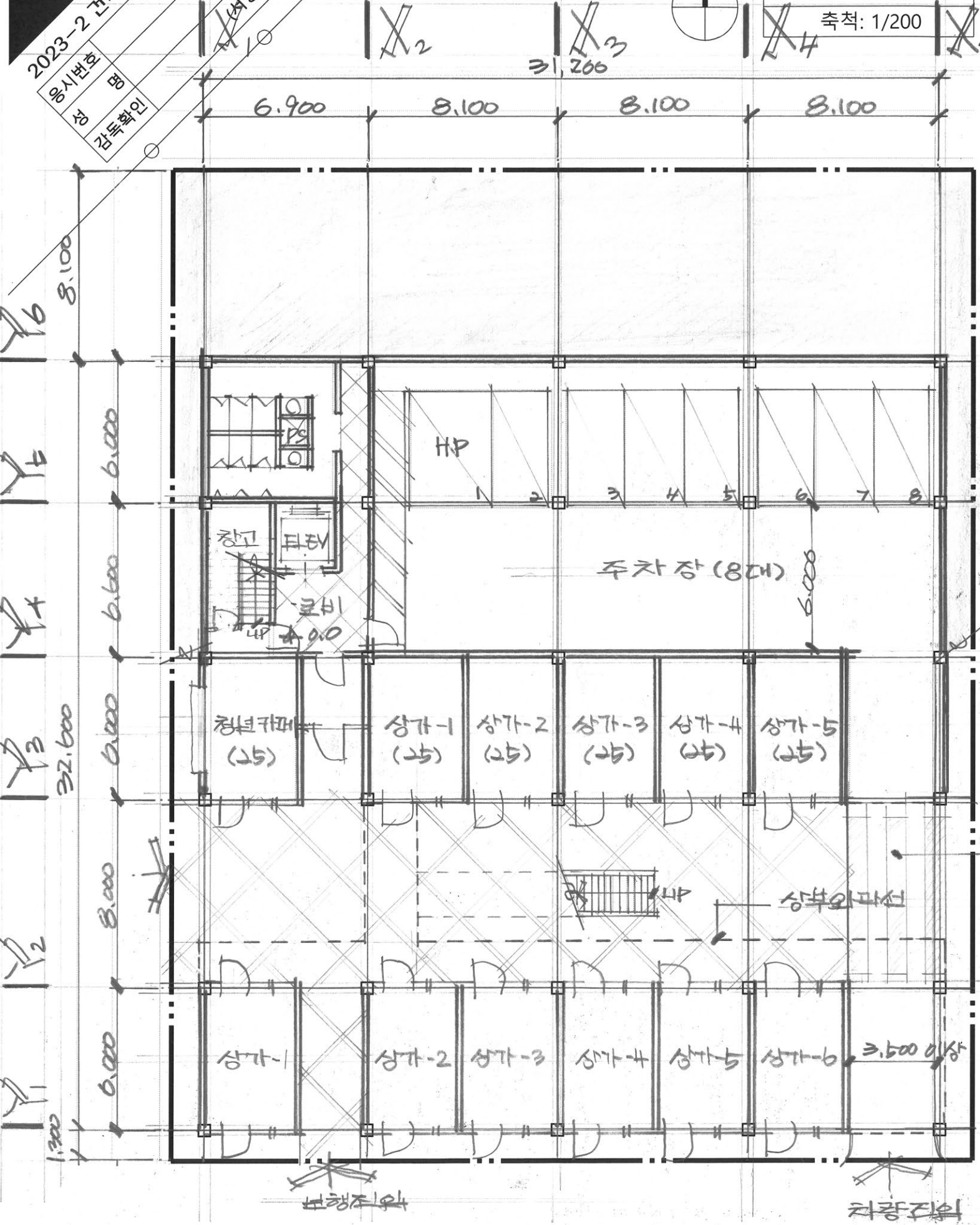
지상 1층 평면도
