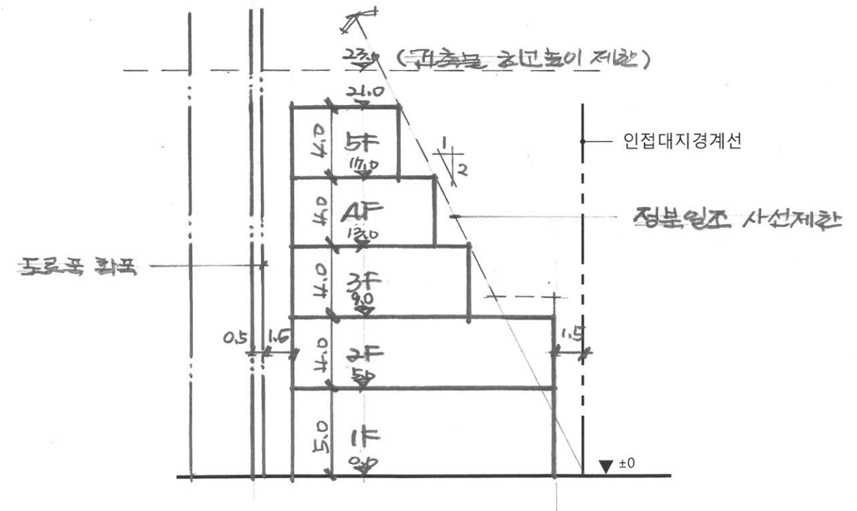
A-A' 단면도 축척: 1/300
