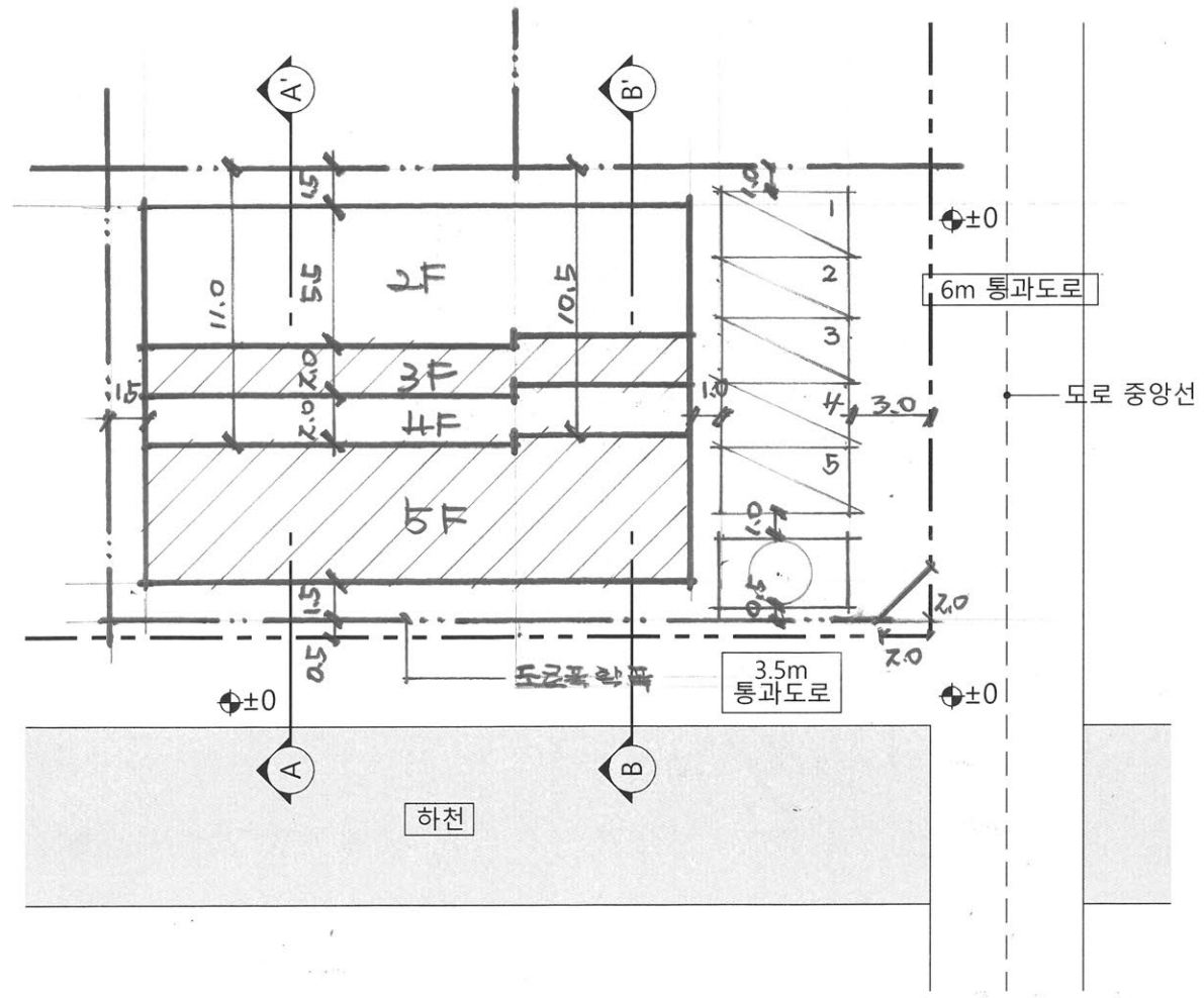
배치도 축척: 1/300
