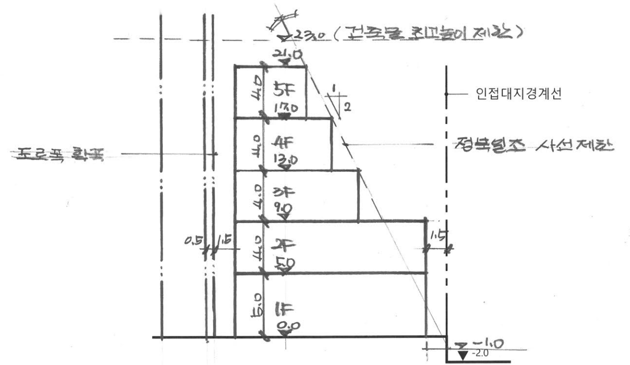
A-A' 단면도 축척: 1/300
