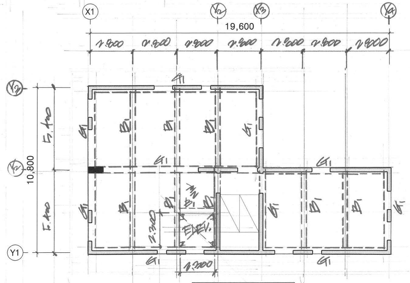
지상 3층 구조평면도 축척: 1/150
