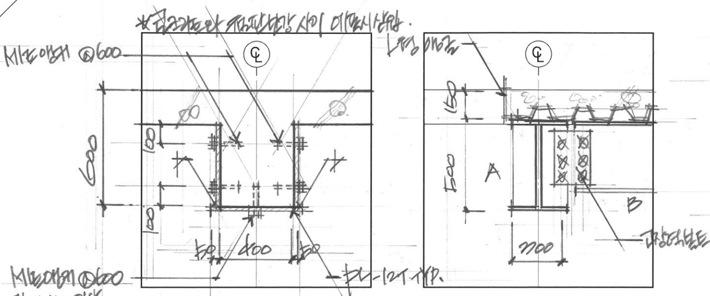
구조보강 단면상세도 축척: 1/20
