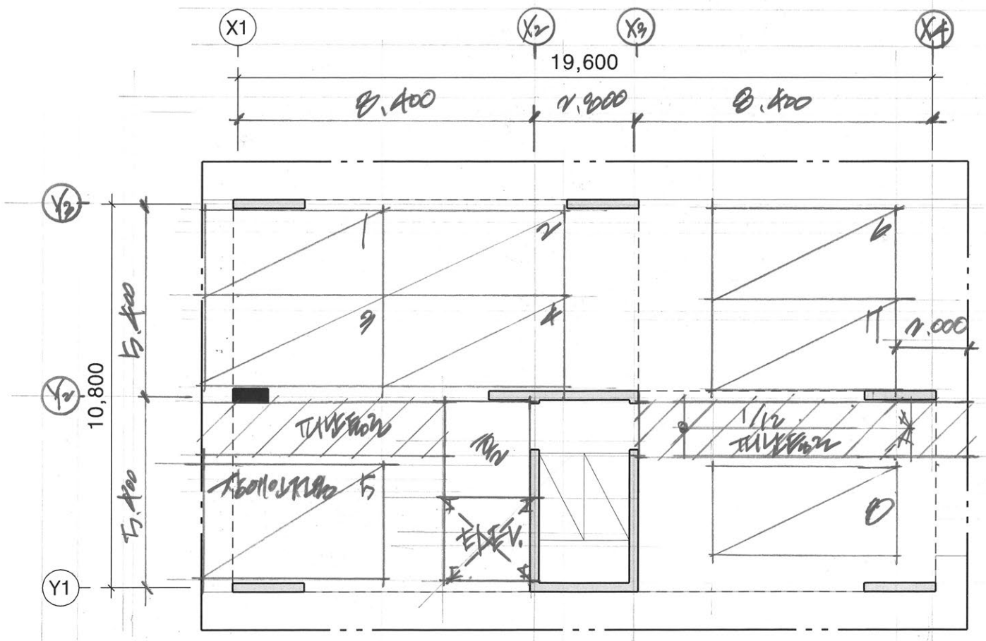
지상 1층 평면도 축척: 1/150
